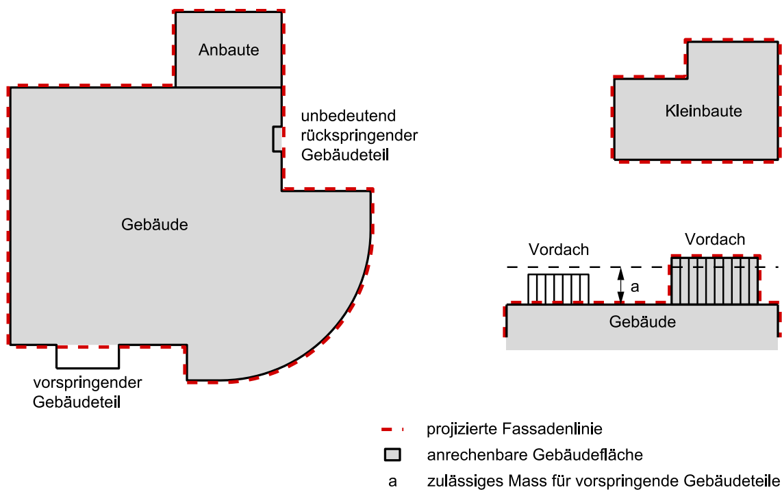
Figur 8.4 Anrechenbare Gebäudefläche
